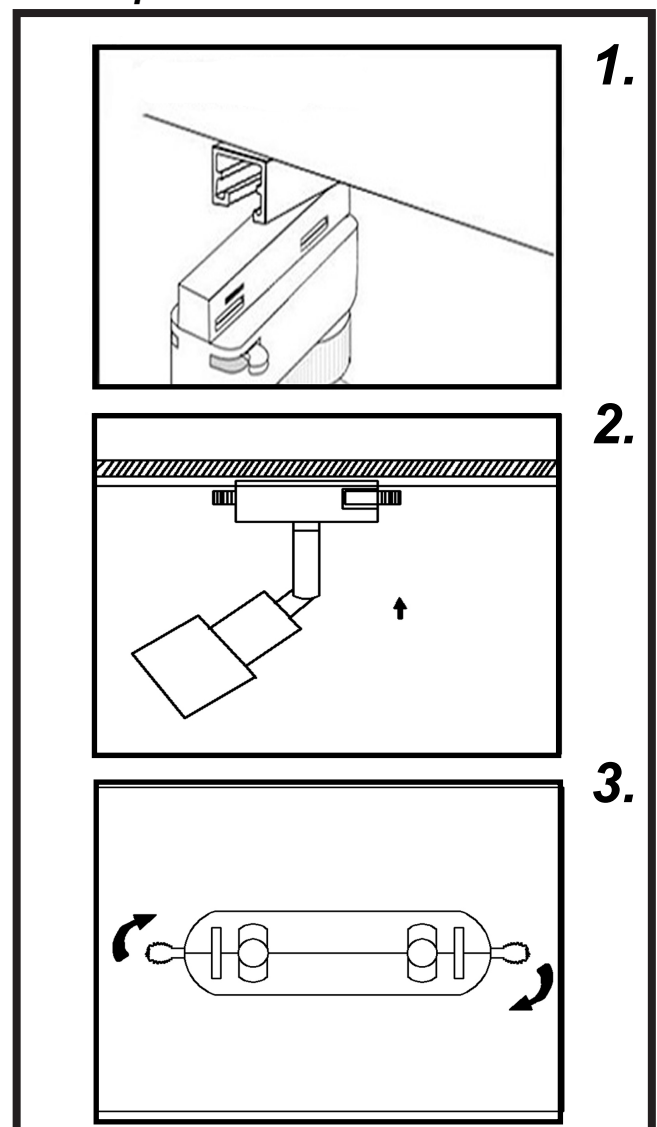
Схема установки трекового светильника.
